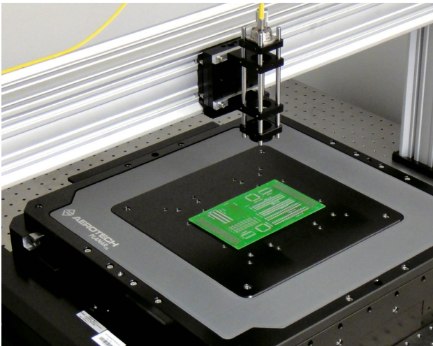
Fertigungseinrichtung zur Direktbelichtung von lichtempfindlichen Schichten mittels UV-Laserstrahl.
