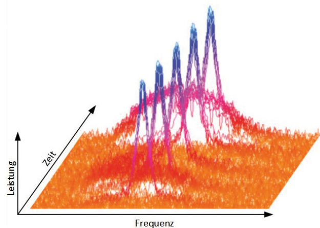
Spektrales Messergebnis experimenteller Untersuchungen im 2,4 GHz-Frequenzband
