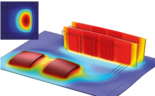
kleines Bild: Intensitätsprofil in einem gekrümmten Wellenleiter, großen Bild: Statische Lösung des thermomechanischen Modells einer Leiterplatte mit jeweils zwei passiv gekühlten Prozessoren und Speichermodulen die jeweils 80 W bzw. 20 W dissipieren (Kühlkörper sind nicht dargestellt).
