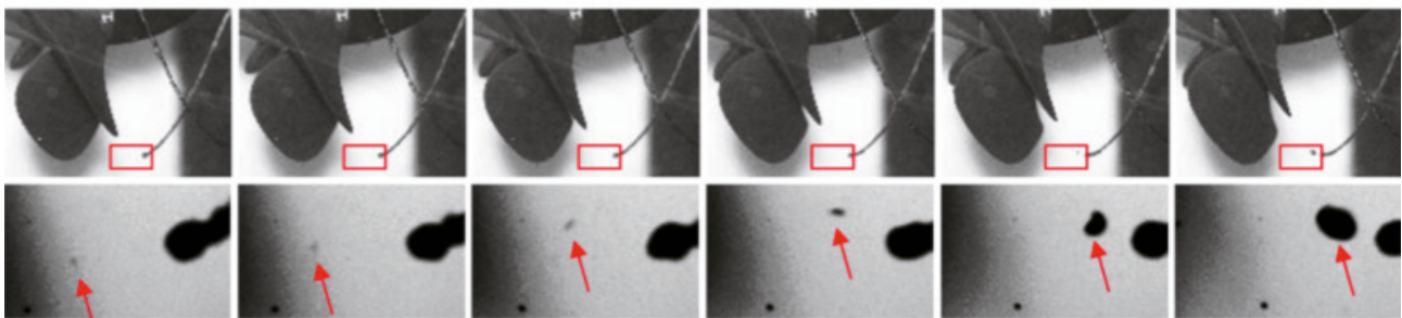
Auftreten der Spitzenwirbelkavitation durch Keime in der Propellerzuströmung. Die Hydrodynamic Nuclei Concentration Technik ermöglicht eine schnelle und statistisch sichere Bestimmung der Keimkonzentration.
