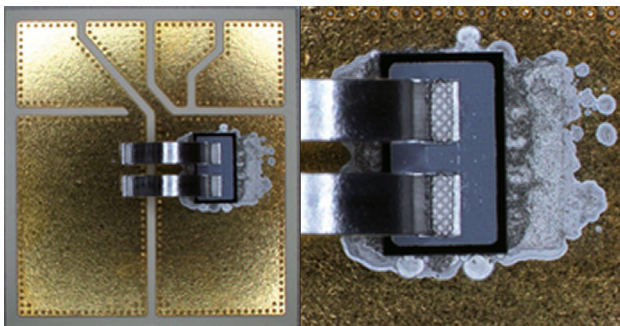
Power-MOSFET mit temperaturstabiler Lötverbindung auf DCB-Keramiksubstrat gelötet, Al-Bändchen als Oberseitenkontakt (Foto: A. Fix, Bosch)
