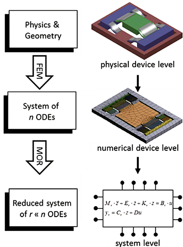
Modelordnungsreduktion Design Flow
