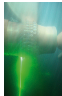
Abb: Modellpropeller mit Luftblasen im Kavitationstunnel (links) und Lasermesstechnik am realer Schiffspropeller (rechts)
