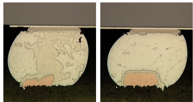
Abb. 2: Lötverbindungen (2,5 A nach 600 h)
