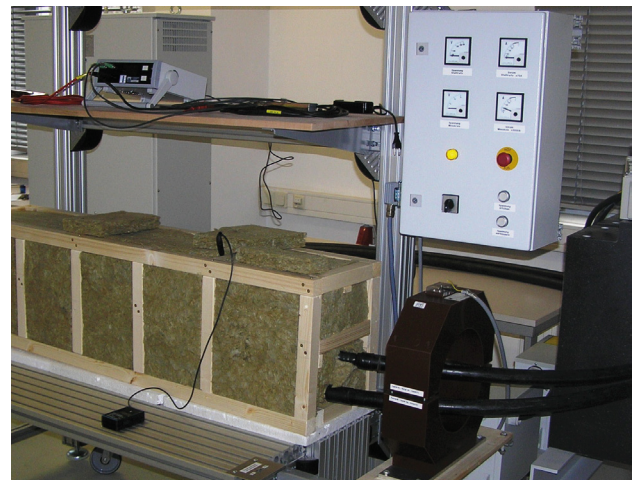
Abb. 2: Hochstrom-Versuchsstand
